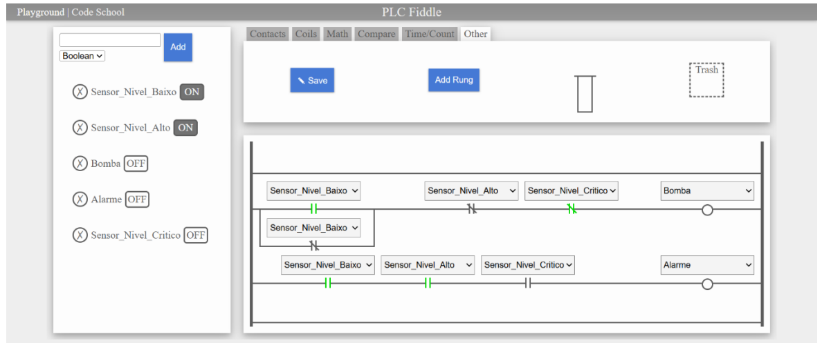
Figura 4 - Sistema em condição de nível máximo
